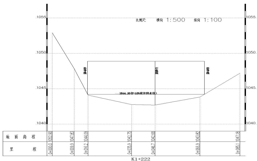
图 5-1 实测断面
