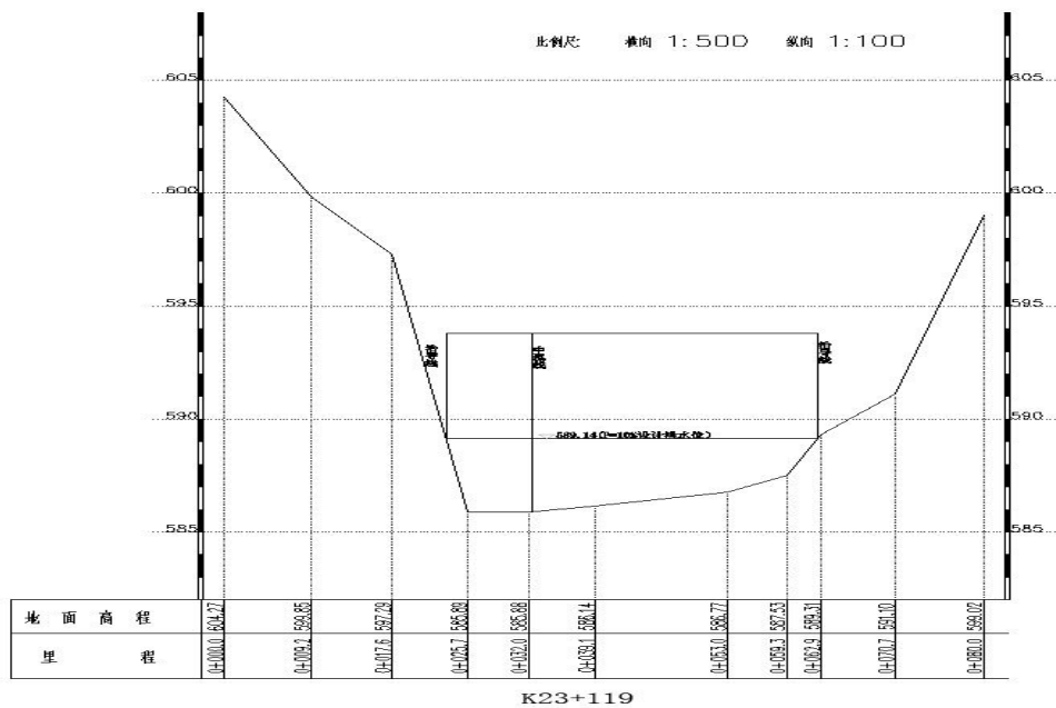
图 5-3 现状实测断面
