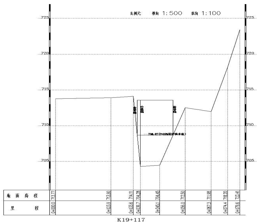
图 5-2 现状实测断面
